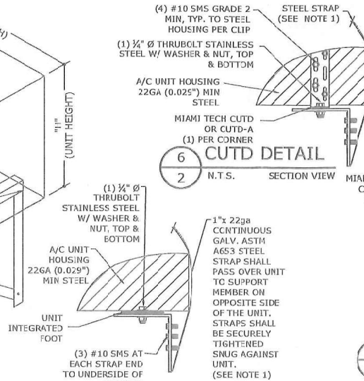
5 STRAP DETAIL N.T.S. SECTION VIEW
